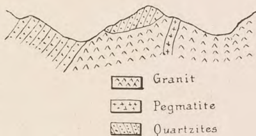
Fig. n° 21. Profil par le gisement de Tétéhina.
