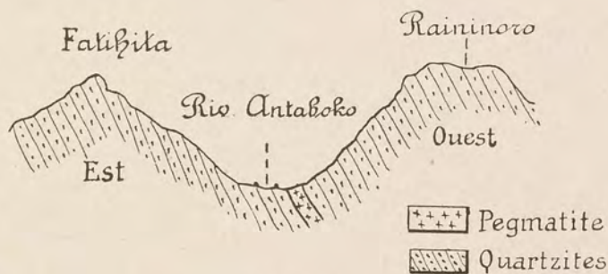
Fig. n° 18. Profil par le gisement d'Antaboko.
